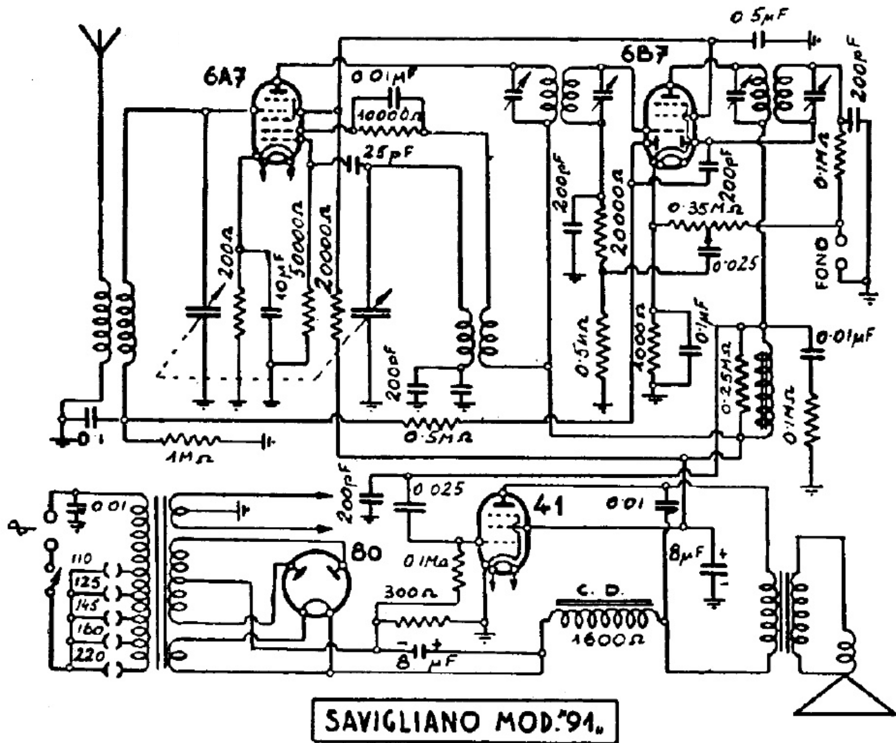
S. A. OFFICINE DI SAVIGLIANO. — Mod. « 91 ». — Produzione 1938. - Media frequenza: 480 kHz.
